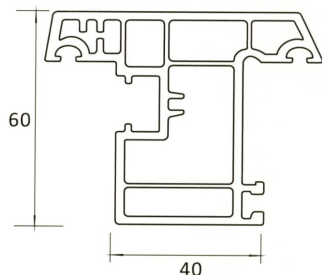
CP 404-B WINDOW SASH B
