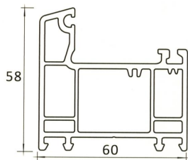
CP 401 MAIN FRAME
