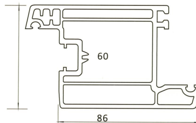
CP 406-B DOOR SASH INTERNAL B
