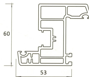
CP 404 WINDOW SASH
