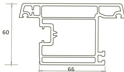
CP 405-B DOOR SASH EXTERNAL B
