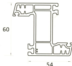
CP 403-C Z-SASH MULLION
