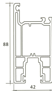
SP 403B 42MM DOOR SASH B
