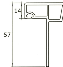
AP419 60 DOOR CONNECTOR
